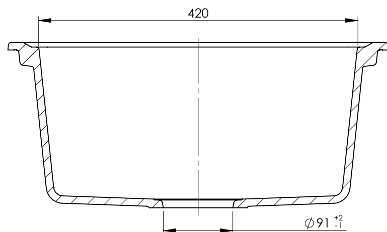
PRZEKRÓJ B-B
